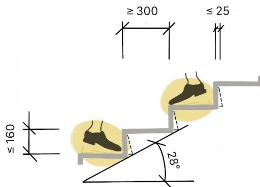
Obrázek 13 – Požadavky na schodišťové stupně
