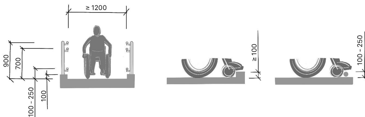
Obrázek 15 – Bezbariérová rampa a minimální parametry
