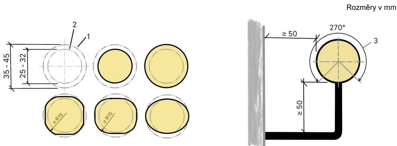
Obrázek 18 – Zábradelní madlo – umístění a tvarové řešení
