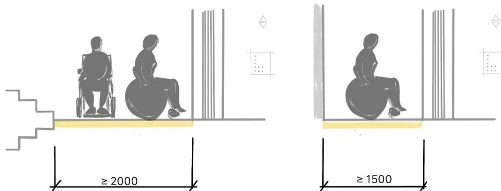
A) Volný prostor nástupního místa navazující na schodiště
